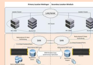
Redundanz Rechenzentrum
